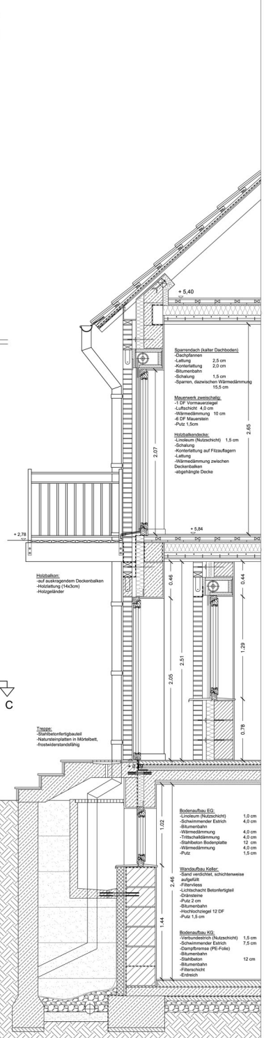
Schnitt B-B
