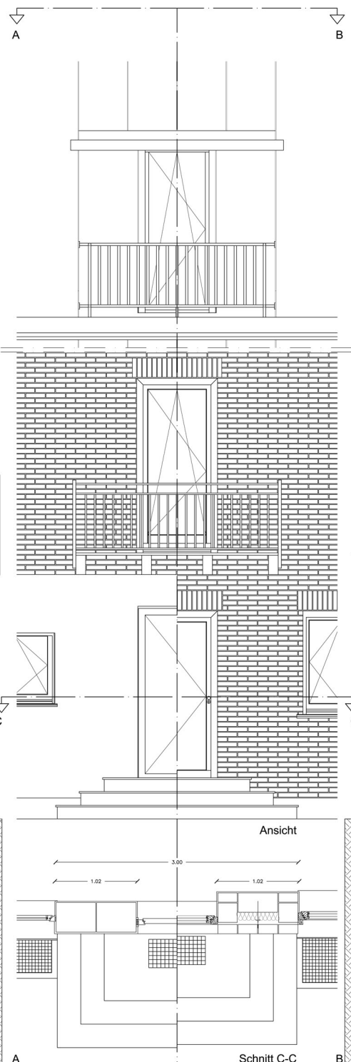
Schnitt C-C
